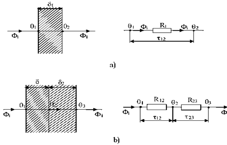
Şəkil 1. Birqat (a) və ikiqat (b) hissələr üçün istilik əvəz sxemləri
