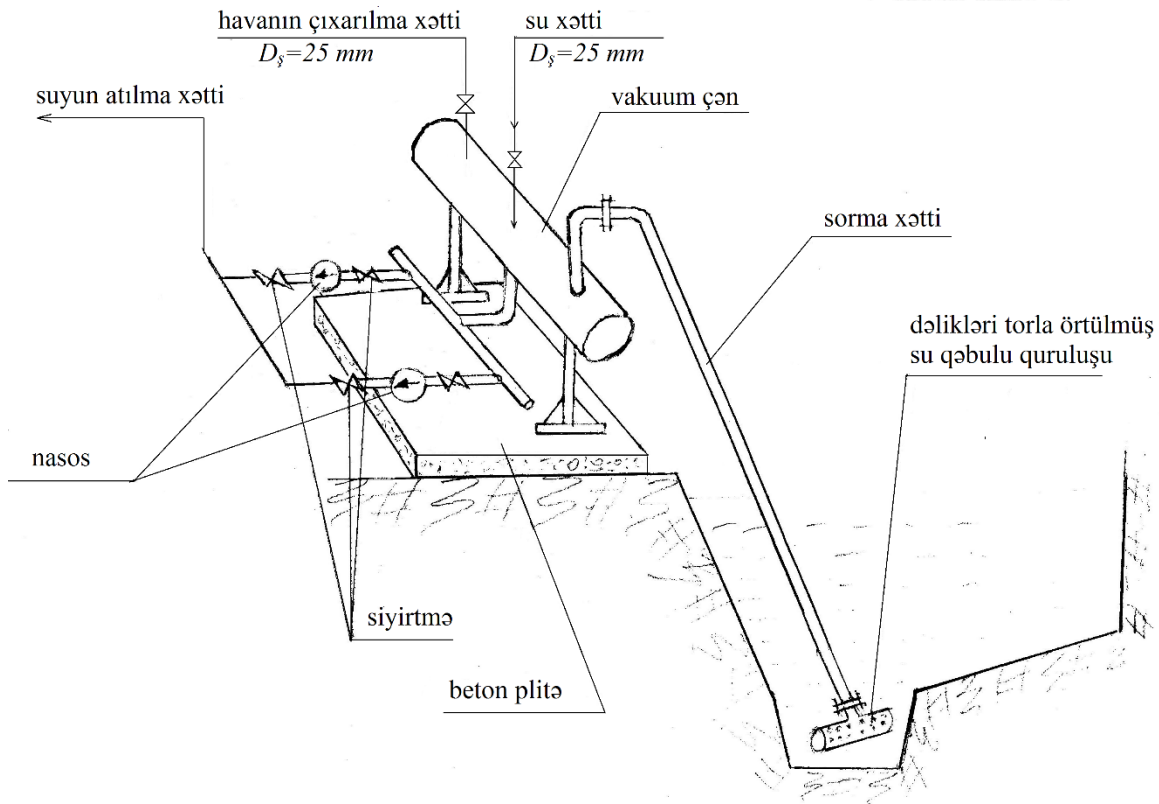
Şəkil 1. Drenaj sularının sorulub atılması sxemi
