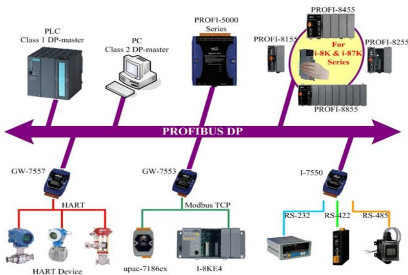
Şəkil 1. Sənaye idarəetmə prosesinin struktur sxemi
