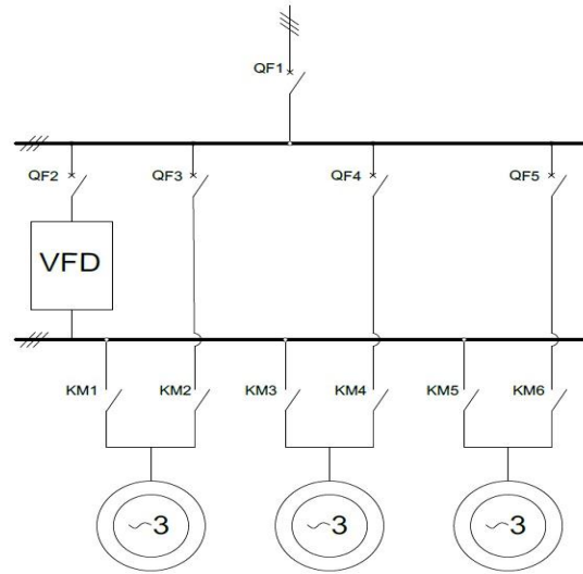
Şəkil 3. Mühərrikin yeni idarəetmə sisteminin birxətli sxemi
