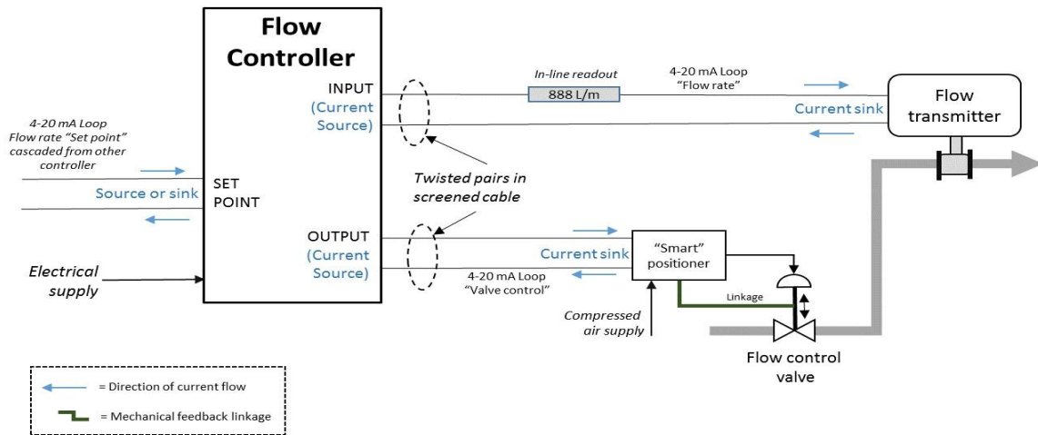
Şəkil 2. MİD tipli tənzimləmənin sxemi
