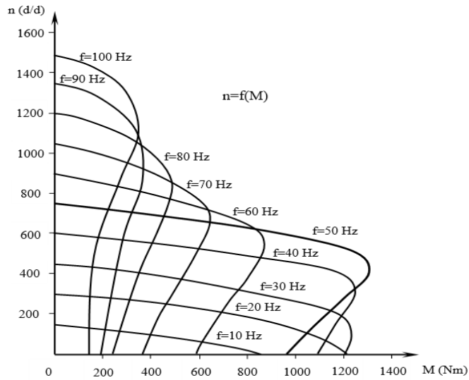
Şəkil 2. MAP 622-4/8/16 tipli AM -in müxtəlif tezliklərdə tənzim xarakteristikaları
