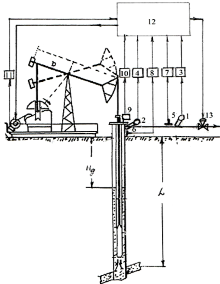
Şəkil 1. Lay mayesinin və qazın debitinin ölçülməsi qurğusunun prinsipial sxemi
