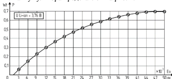
Рис. 4. График P = f(E_{\text{в}}) солнечной батареи при подключении аккумулятора
