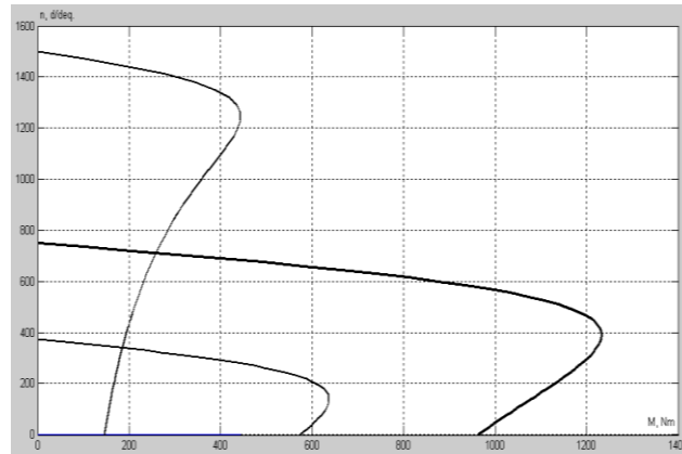
Şəkil 1. MAP 622-4/8/16 tipli AM-in ayrı-ayrı dolaqlarının təbii mexaniki xarakteristikaları
