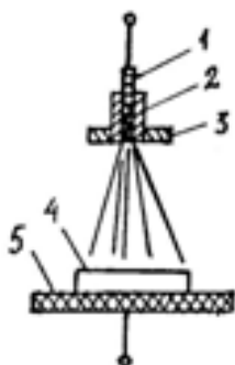
Şəkil 2. Məşəl qazboşalması reaktorunun aktiv elementi
