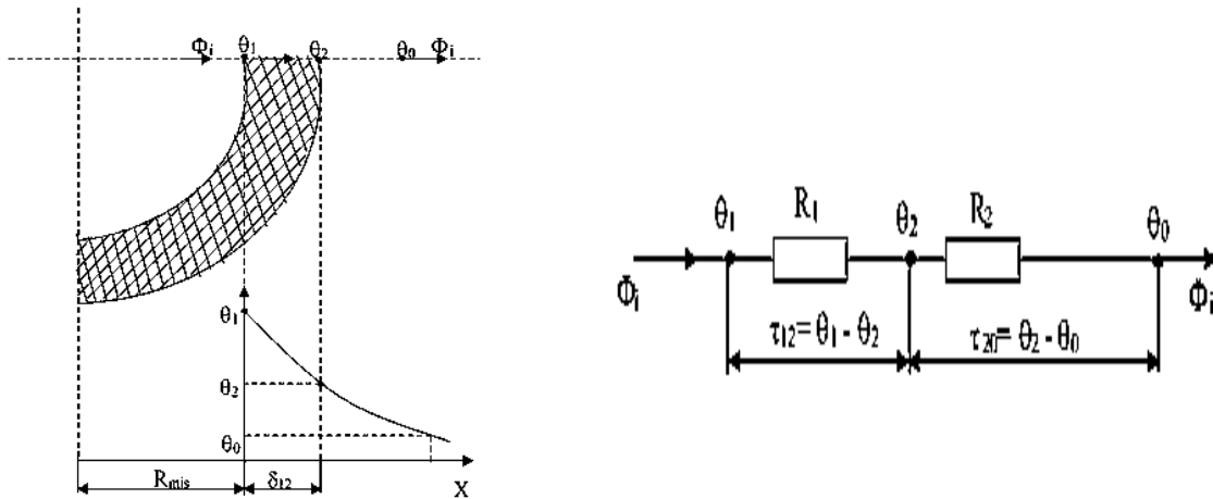
Şəkil 2. İzolyasiyalı naqıl üçün istilik əvəz sxemi
