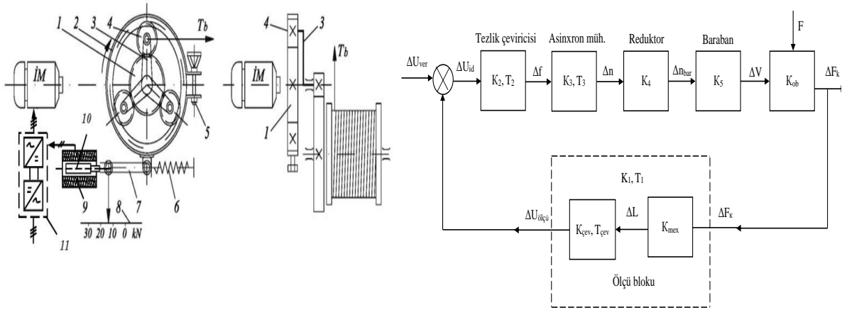
Şəkil 1. Planetar ötürücülü ölçmə qurğusu Şəkil 2. AYB-nin struktur sxemi
