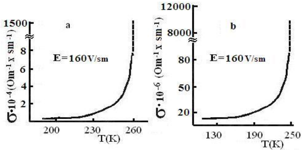
Şəkil 1. TIInTe 2 birləşməsində xüsusi keçiriciliyin temperaturdan asılılığı (a-tetraqonal ox istiqamətində, b- oxa perpendikulyar istiqamətdə)
