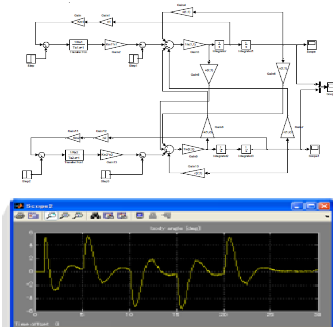
Şəkil 4. Mobil robotun S -modeli və kompüter simulyasiyası
