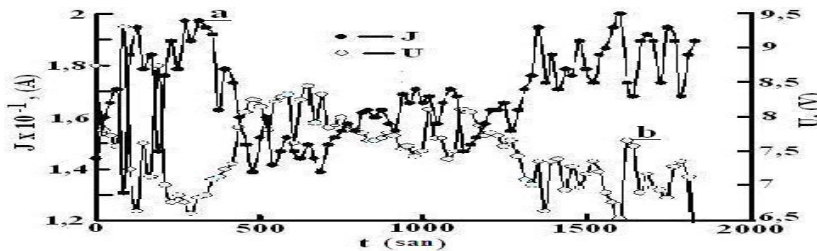
Şəkil 3. TIInTe 2 kristalında cərəyanın və gərginliyin ossilyasiyası (a- cərəyan, b- gərginlik)
