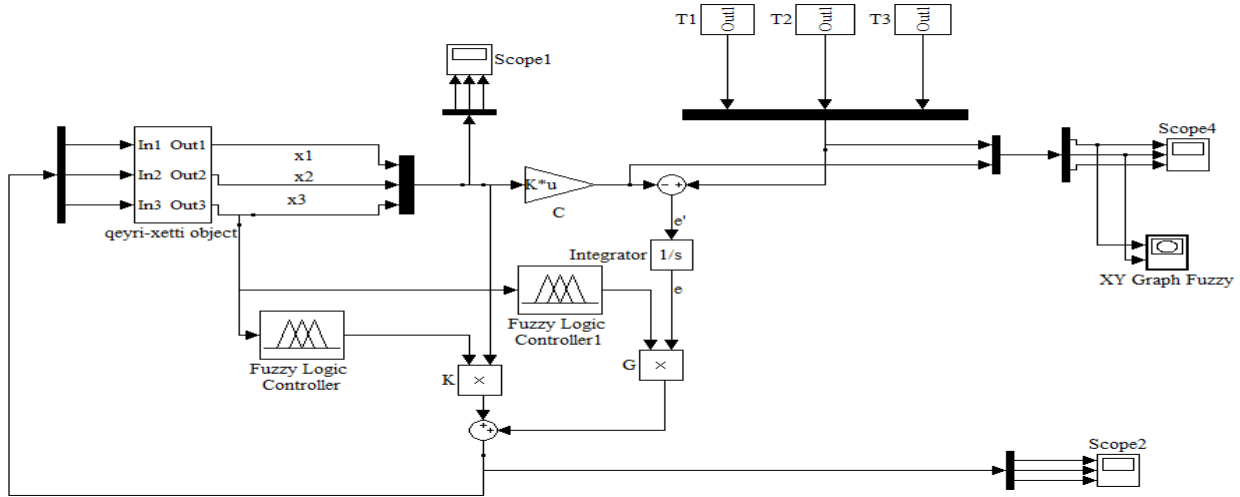
Şəkil 1. Mobil robotun qeyri-səlis idarəetmə sisteminin S- modeli
