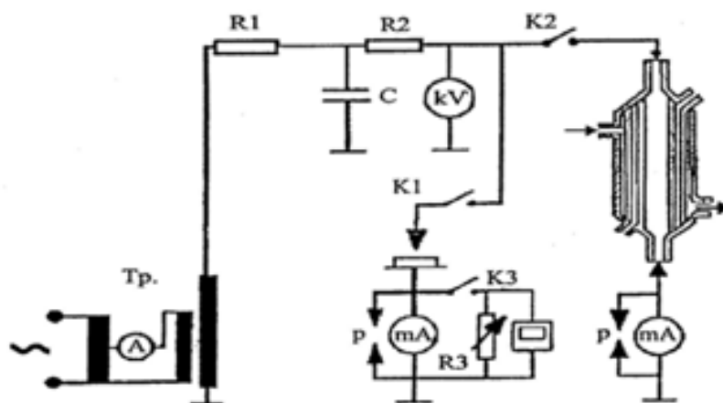
Şəkil 1. Tac və arakəsməli elektrik qazboşalmasının sxemi
