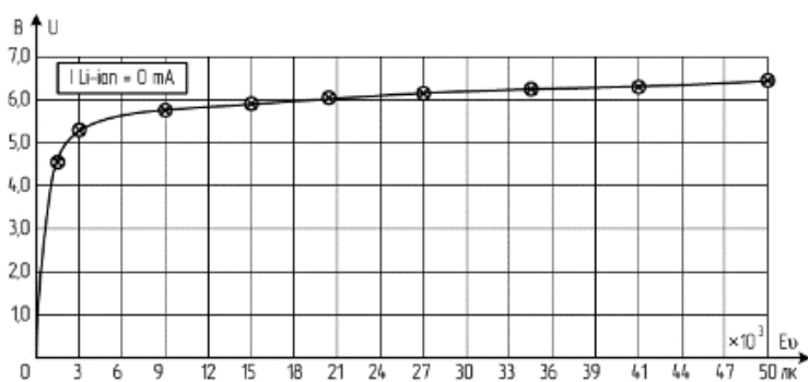
Рис. 2. График U = f(E_{\text{в}}) солнечной батареи без подключения нагрузки
