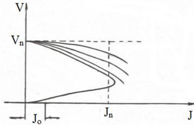
Şəkil 2. Cəryan-gərginlik xarakteristikası
