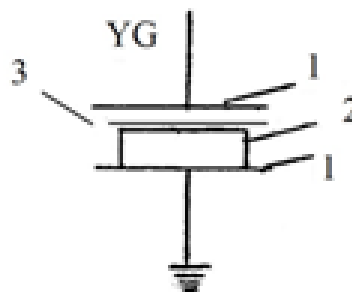
Şəkil 3. Arakəsməli qazboşalması reaktorunun aktiv elementi
