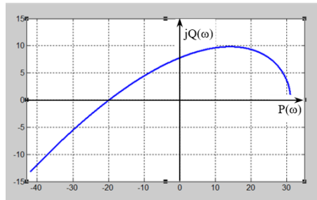
Şəkil 3. Mixaylov hodoqrafı
