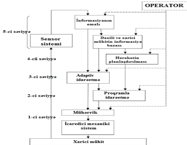
Şəkil 3. Mobil robotun funksional iyerarxik quruluşu
