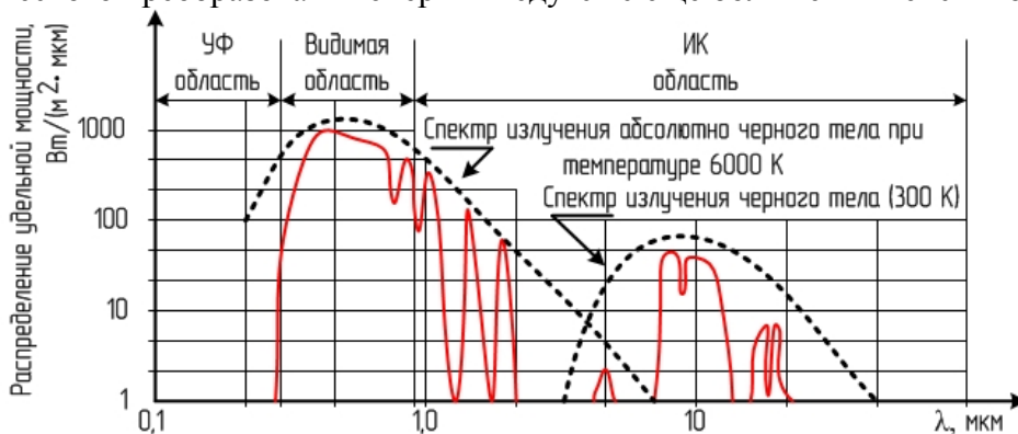
Рис. 1. Зависимость плотности излучения Солнца и земной поверхности от длины волны
