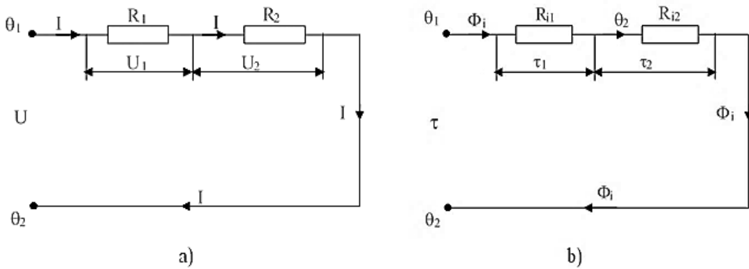
Şəkil 3. Elektrik (a) və istilik (b) dövrlərinin analogiyası
