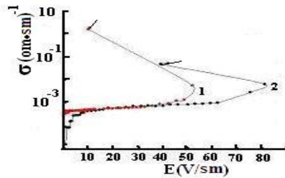
Şəkil 2. TIInTe 2 kristalının T=300K temperaturunda \sigma elektrik keçiriciliyinin E elektrik sahəsinin intensivliyindən asılılığı: əyri 1– kristalın tetraqonal c oxu istiqamətində ölçmə, 2 – c oxuna perpendikulyar istiqamətində
