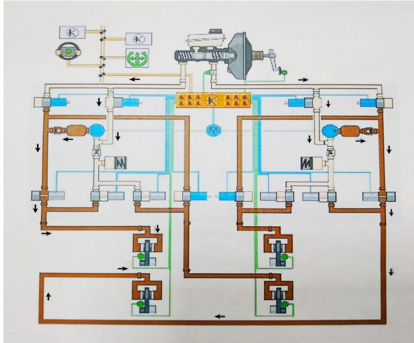
Şəkil 1. Minik avtomobillərində dinamik stabilləşdirmə sistemi
