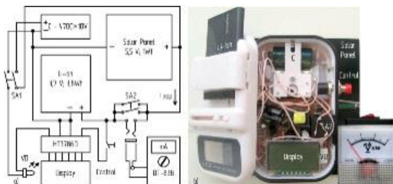
Рис. 3. Структурная схема (а) и внешний вид (б) зарядного устройства «Фотон»
