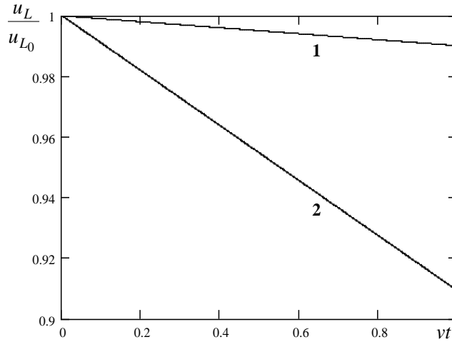
Şəkil 1. Çubuğun yuxarı ucunun u_L/u_{L_0} yerdəyişməsinin vt zamandan asılılığı:
