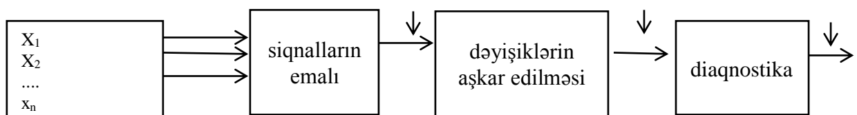
Şəkil 2. Texniki diaqnostikanın funksional sxemi
