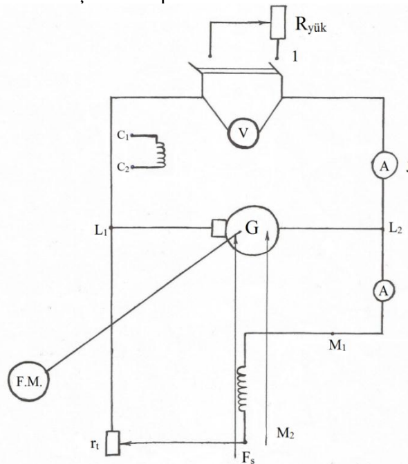
Şəkil 1. Öz-özünə təsirlənmə rejimində ardıcıl dolağı birləşdirmədən generatorun xarici xarakteristikası
