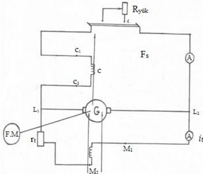
Şəkil 3. Öz-özünə təsirlənmə rejimində ardıcıl dolaqları paralel dolaq ilə uyğun birləşdirilmiş generatorun xarici xarakteristikası
